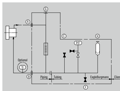
Funktions- und Installationsschema SPO, Plan 53B
